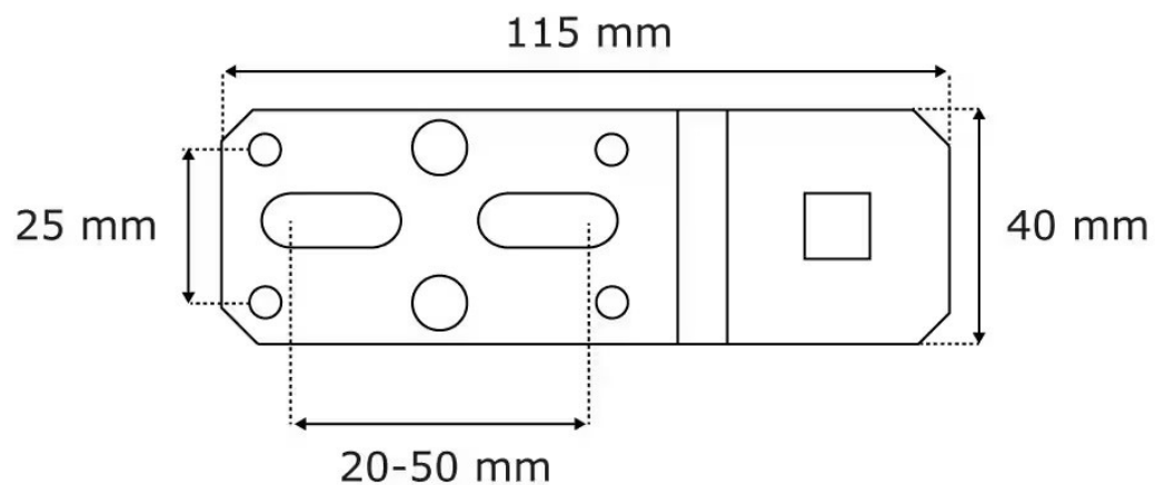
Łożysko płaskie silnika z kołkiemdzielonym (tylko JM45)
