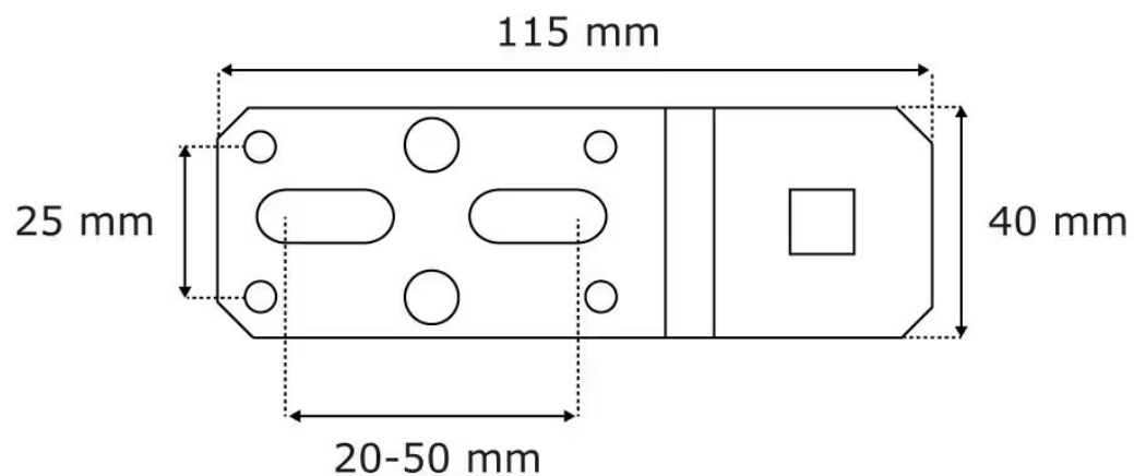
Łożysko płaskie silnika z kołkiem dzielonym (tylko JM45)
