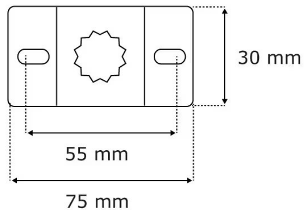
Łożysko gwiazdowe silnika
