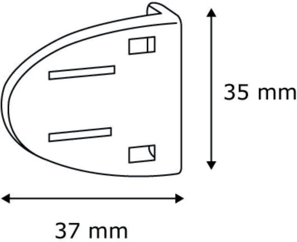
Uchwyt boczny
