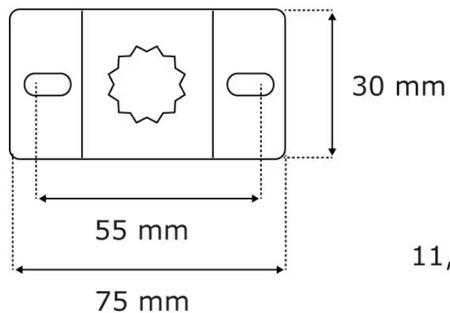
Łożysko gwiazdowe silnika
