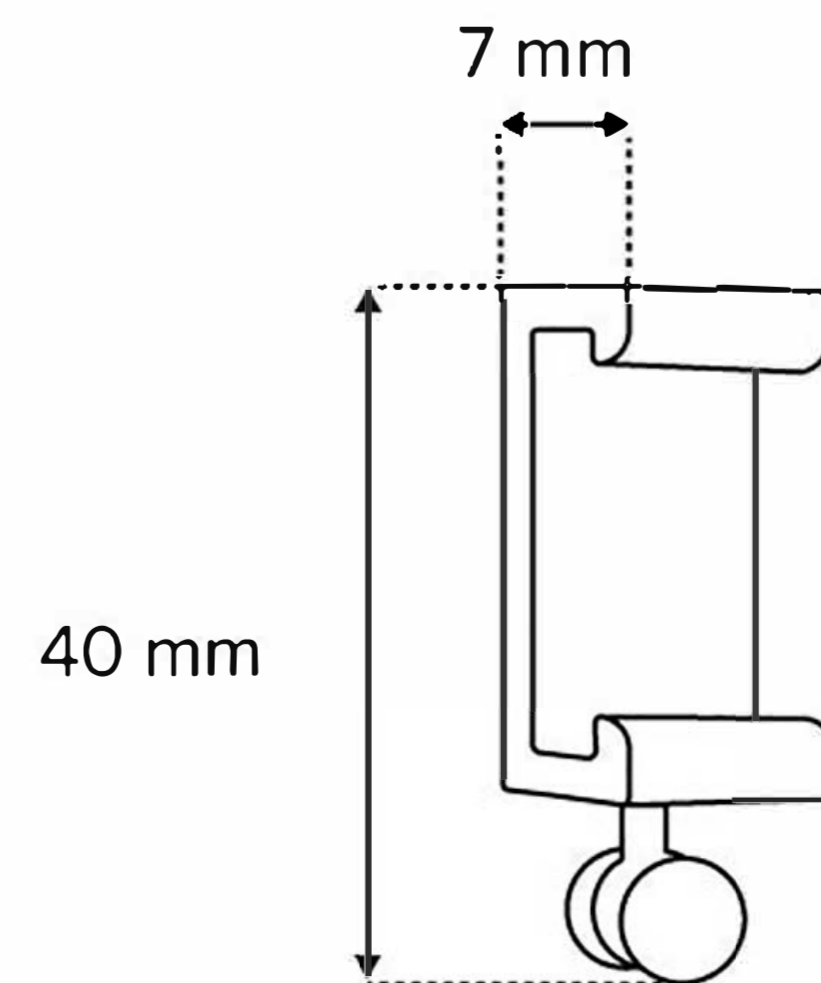
3x Ślizgacz kulkowy
