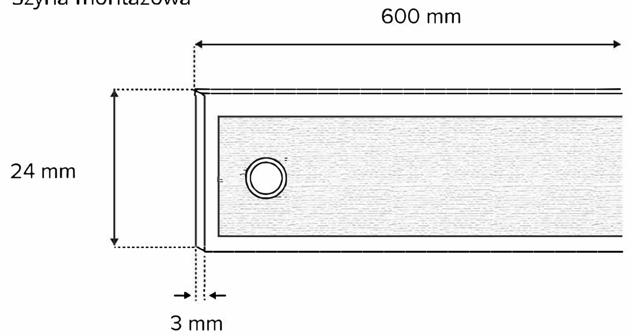
Szyna montażowa
