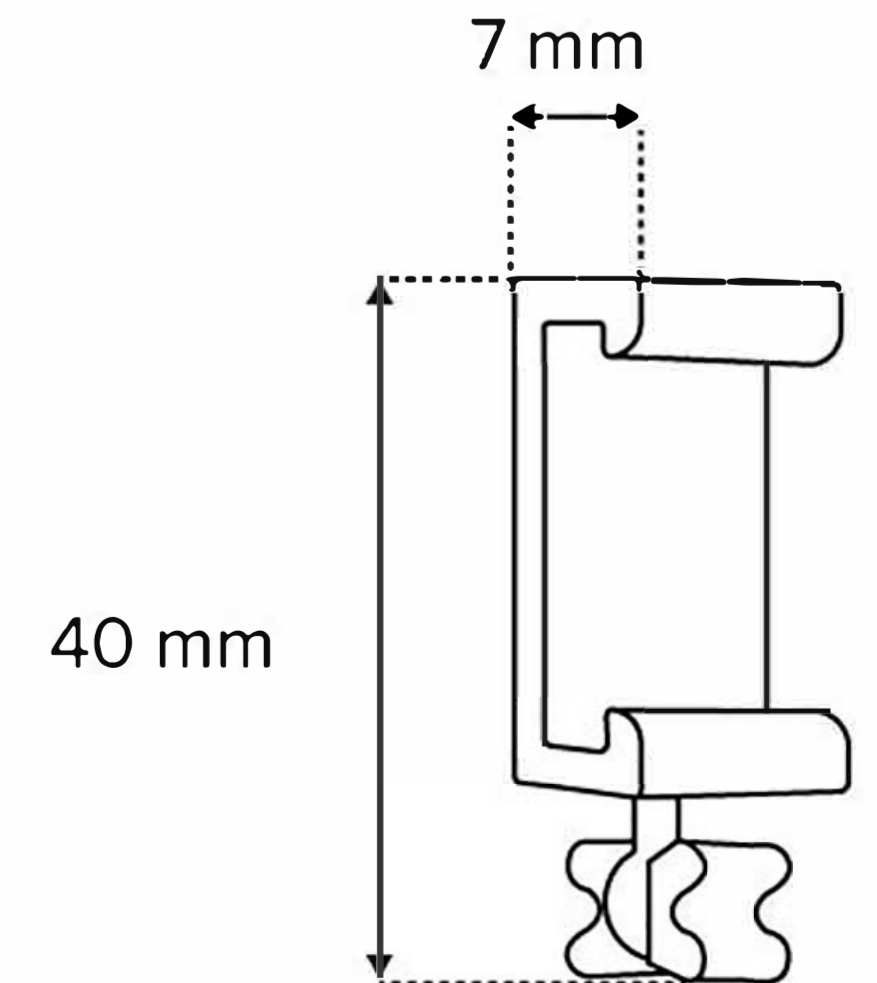
3x Ślizgacz typu X
